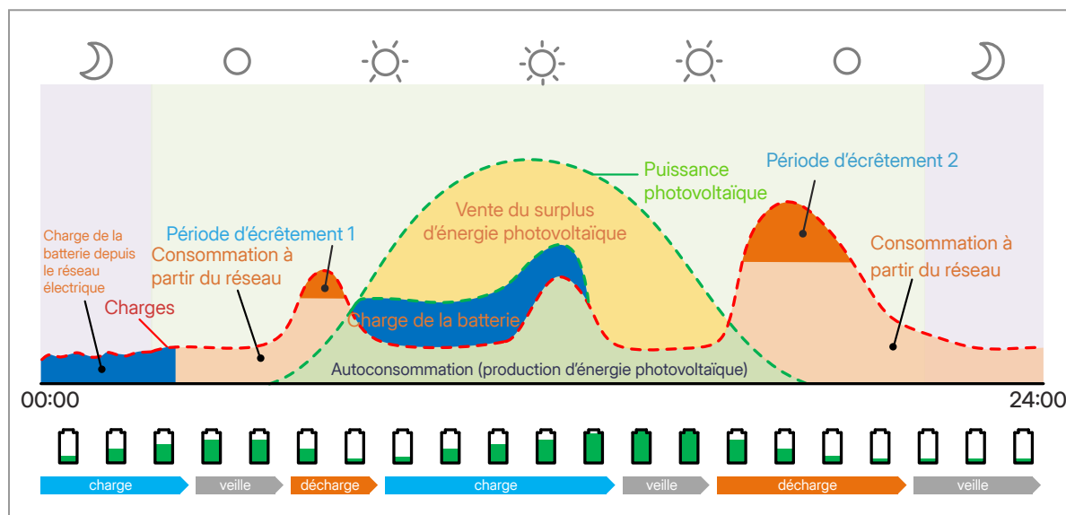
Figure 4-10 Flux de puissance en mode écrêtement
